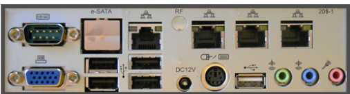
VERSIONE 4 ETHERNET – 1 SERIALI
