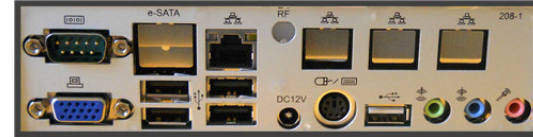
VERSIONE STANDARD o THIN CLIENT
