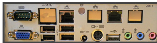
VERSIONE 2 ETHERNET – 1 SERIALE
